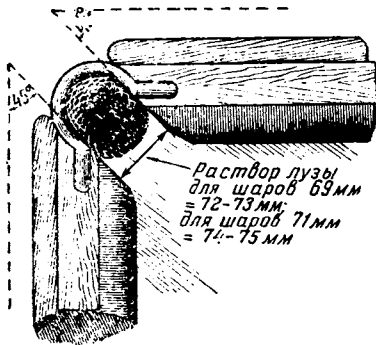
Рис. 32. Устройство угловой лузы.
